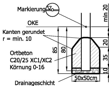
Fundamentschnitt Robinenerdeinbau
