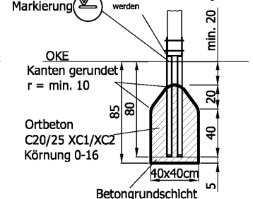
Fundamentschnitt Pfostenschuheinbau F60x800 bei 2 Standfüßen von OKE bis zum Pfosten muss ein Freiraum von min. 5cm eingehalten werden
