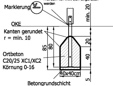
Fundamentschnitt 1/2 Pfostenschuheinbau F60x800 bei 4 Standfüßen von OKE bis zum Pfosten muss ein Freiraum von min. 5cm eingehalten werden
