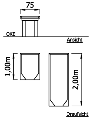
Matschrinnen mit Engpass 09 2947/1 09 2947/2
