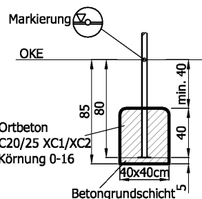
Fundamentschnitt Stahlrohrstützeinbau Art.-Nr.: 15 4067V
